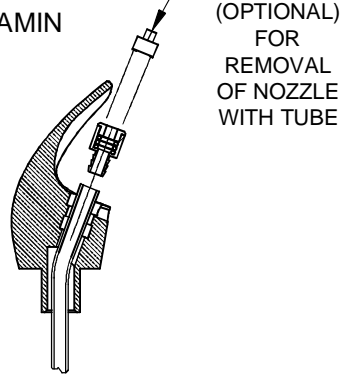
STYLE B (TUBING CONNECTS TO INSERT ASSY)
